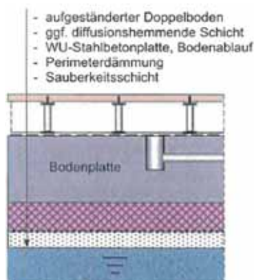
Bild 6 Aufgeständerter Doppelboden, Beanspruchungskategorie 1
