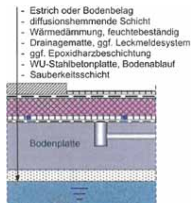
Bild 7 Bodenaufbau mit Drainage, Beanspruchungskategorie 1
